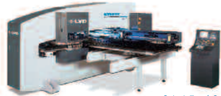
Strippit Σειρά S Διατρητικό μηχανήμα CNC 20 τόνων, υψηλής αποδοτικότητας με πύργο που αποτελείται από 31 σταθμούς.
