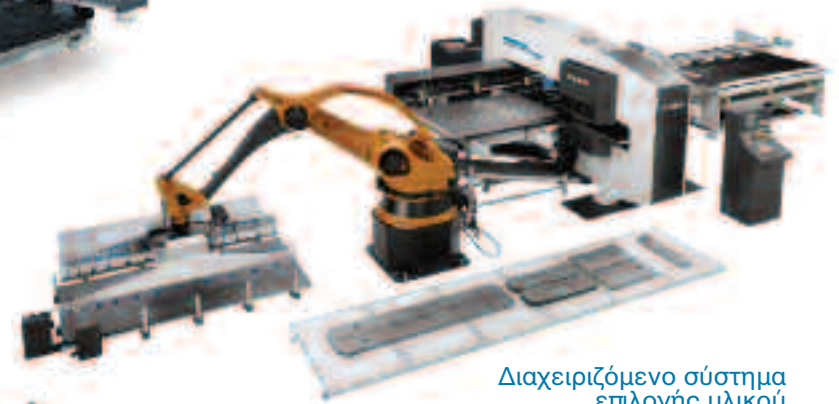
Strippit Σειρά V Μηχανήματα υψηλής αποδοτικότητας, πλήρως εξοπλισμένα, τα οποία συνδυάζουν την δυνατότητα του μεγάλου πύργου με μεγάλες ικανότητες διαμόρφωσης. Είναι διαθέσιμα σε μοντέλα 20 και 30 τόνων.
