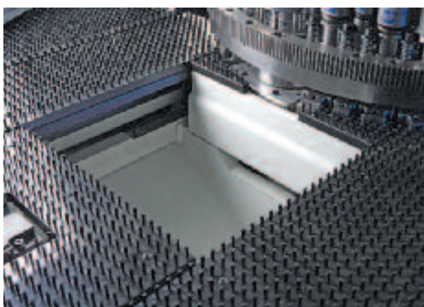
Trappe programmable d'évacuation des pièces de dimensions maxi 500 x 450 mm.
